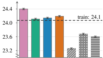
(b) HPSv2
